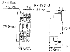
外形圖 (OUTLINE)
