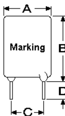
RB 300-30 ~ RB 900-30
