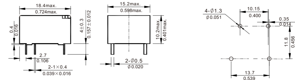
Dimensions
